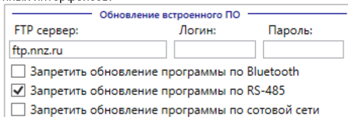
Рис.20. ПО «АСТ Конфигуратор» (OC Windows). Настройка обновления встроенного ПО терминала
