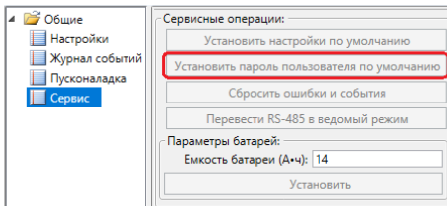
Рис.19. ПО «АСТ Конфигуратор» (OC Windows). Сброс пароля пользователя к заводским настройкам
