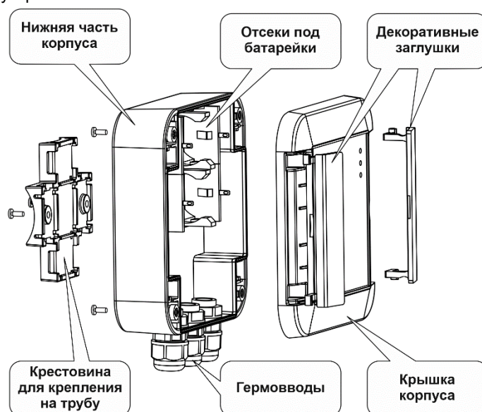
Рис.1. Конструкция терминала
