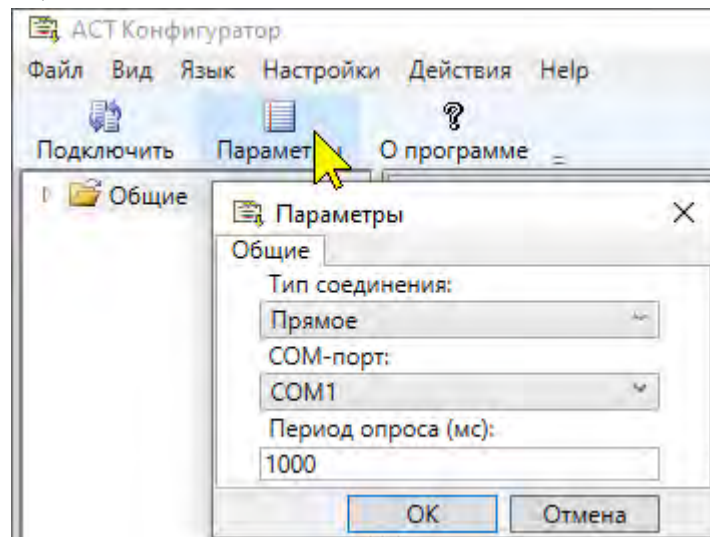
Рис.6. ПО «АСТ Конфигуратор» (ОС Windows). Выбор типа соединения
