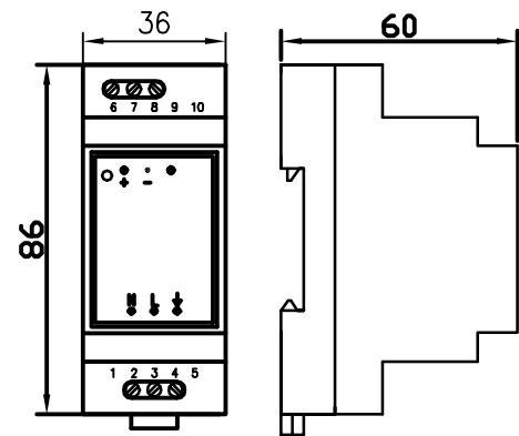
Рис. 1 - Габаритный чертеж
