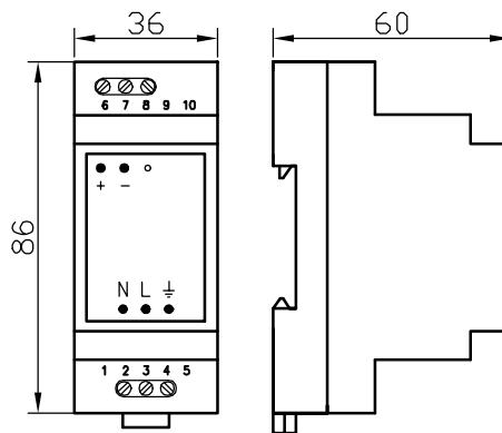
Рис. 1 - Габаритный чертеж
