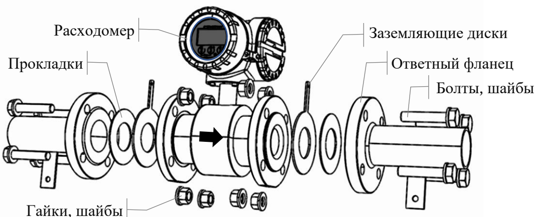
Рисунок 2.6 Установка расходомера
