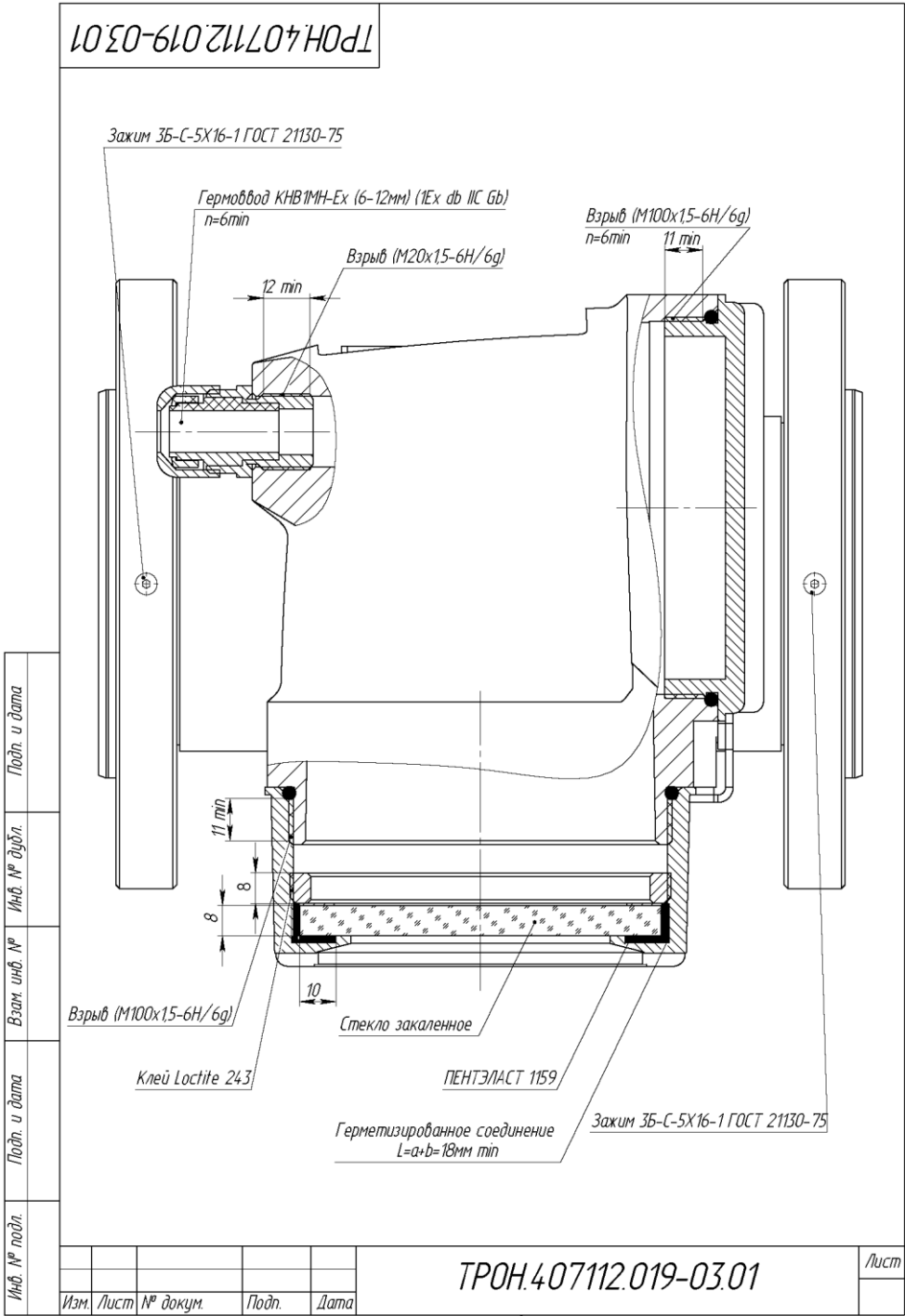
Рисунок Б.2 Взрывонепроницаемая оболочка ("d"). Вид сверху
