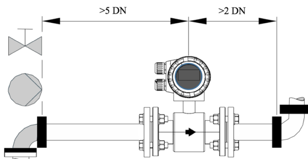
Рисунок 2.3 Длины прямых участков
