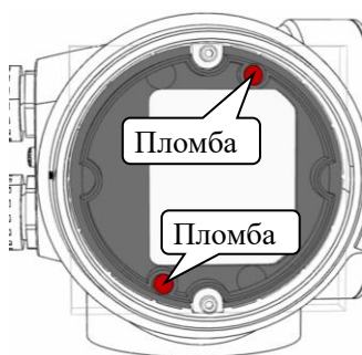
Рисунок 1.5 Пломбирование доступа к изменению метрологически значимых параметров
