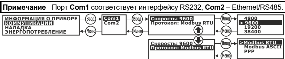
Рис. 3.13 – Настройка Com-портов
